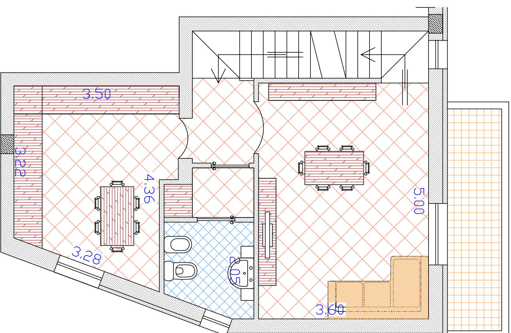
Piano primo
